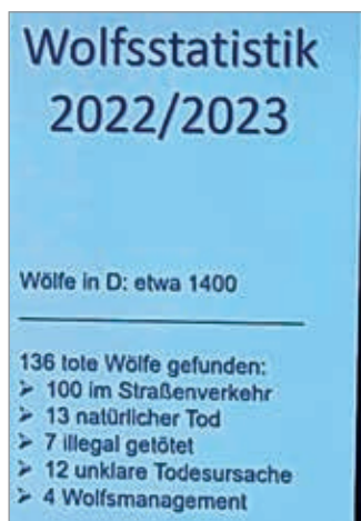
Statistik
