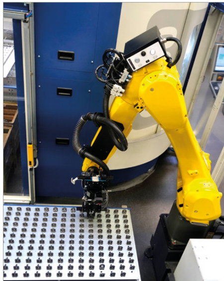
Transformation bei RUD: Automatisierung in der Produktion.
